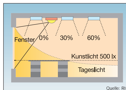
Bild 7 Einzelraumregelung. Erfasst wird die Leuchtdichte des Fensters
